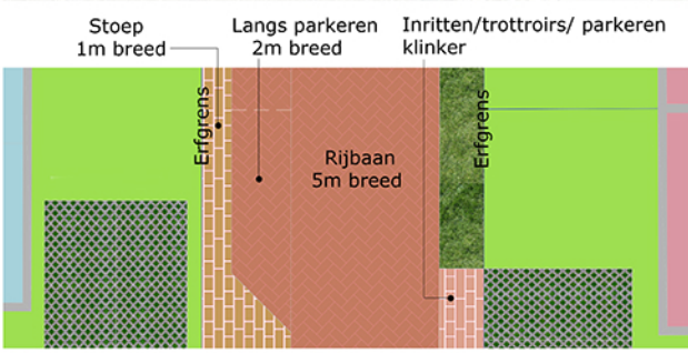
DETAIL PRINCIPLE WEGPROFIEL Schaal: 1:100
